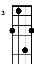
Fmaj7
